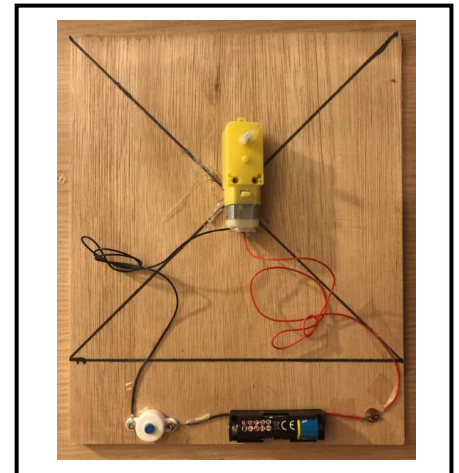
schakelplan
